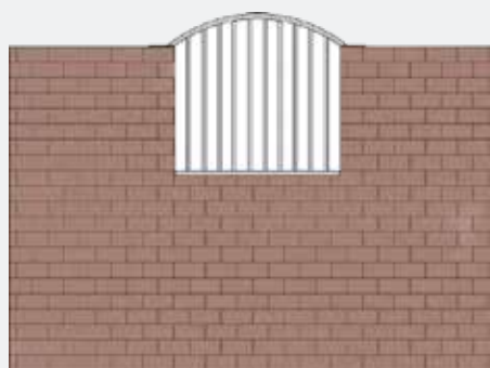
10. Murad mellanvägg med valvat inmurningsgaller.
